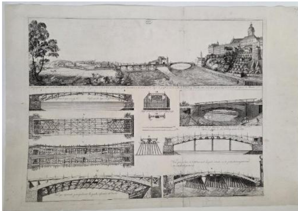
Konstruktion der hölzernen Donaubrücke, Kupferstich von 1811 (Foto: Monika Schierl)
