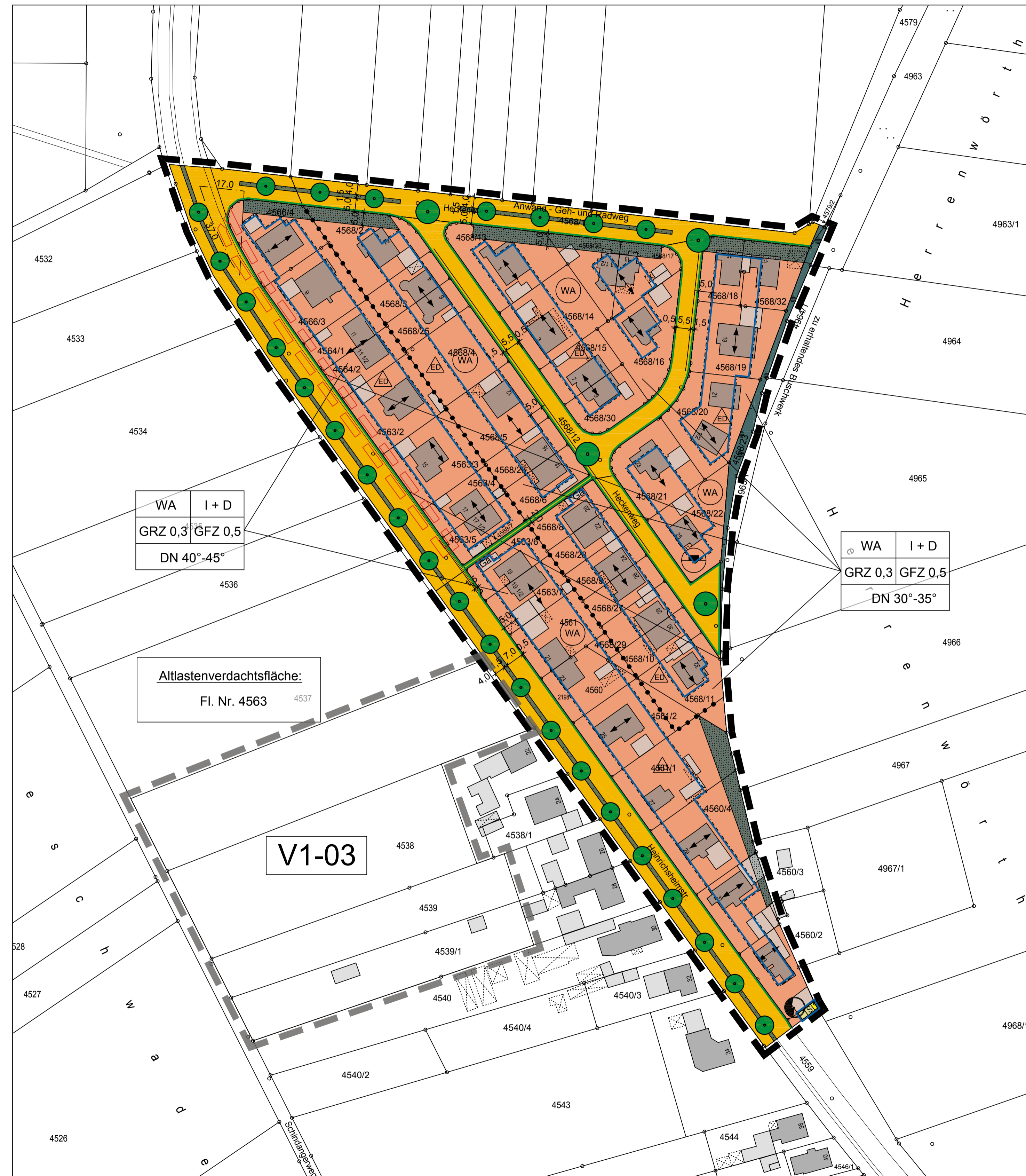
Bebauungsplan "An der Heinrichsheimstraße"
